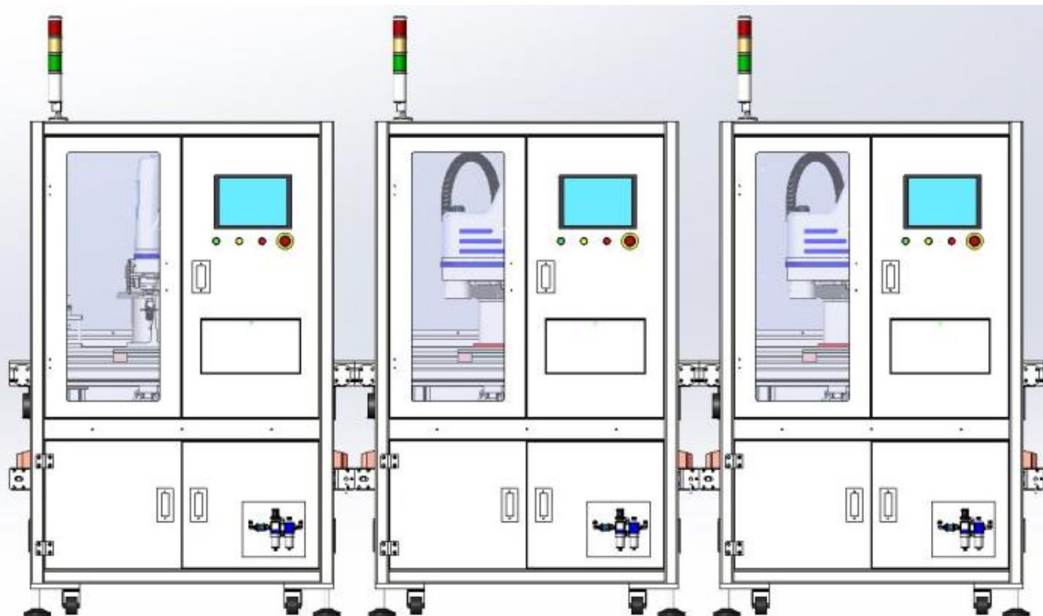
工作区域: 宽400mm, 深350mm, 高120mm Working area: 400 mm (W) × 350 mm (D) × 120 mm (H)
