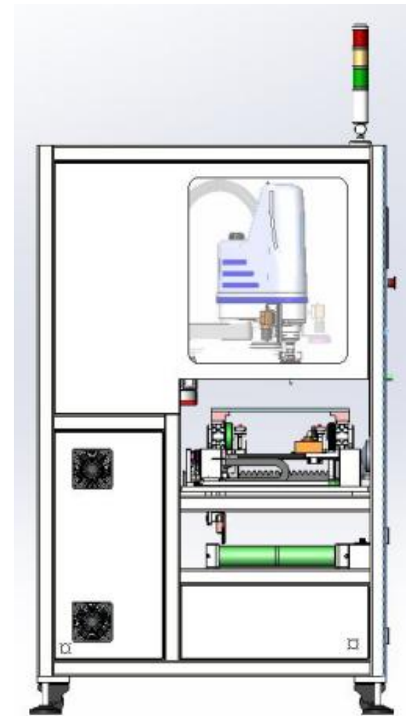
外形尺寸: 宽1000mm, 深1000, 高1800 Overall dimensions: 1000 mm (W) × 1000 mm (D) × 1800 mm (H)
