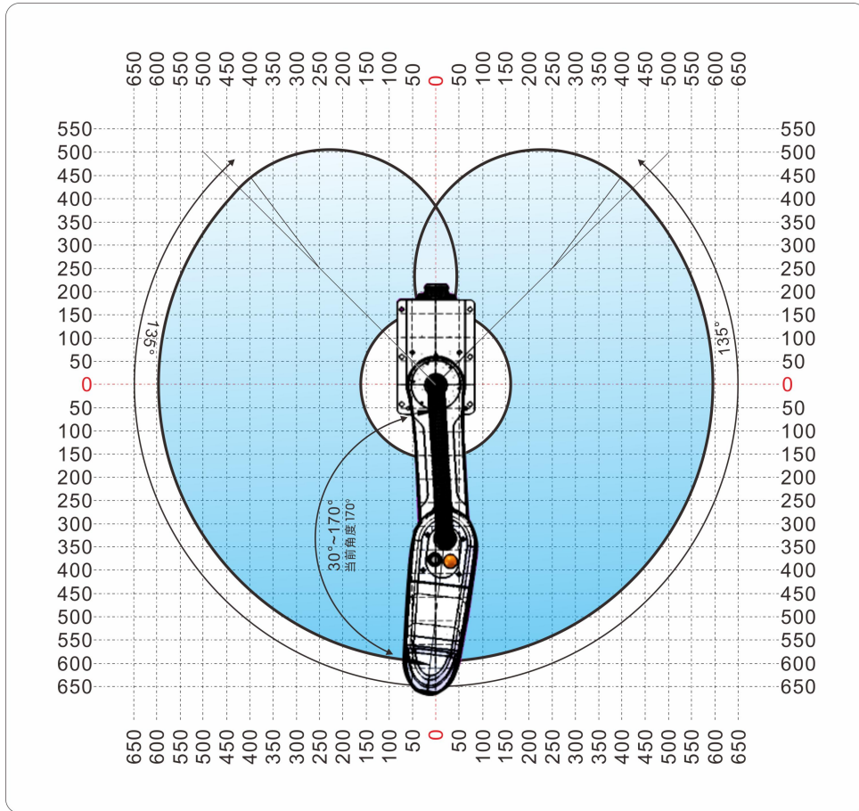
600mm臂展行程图
