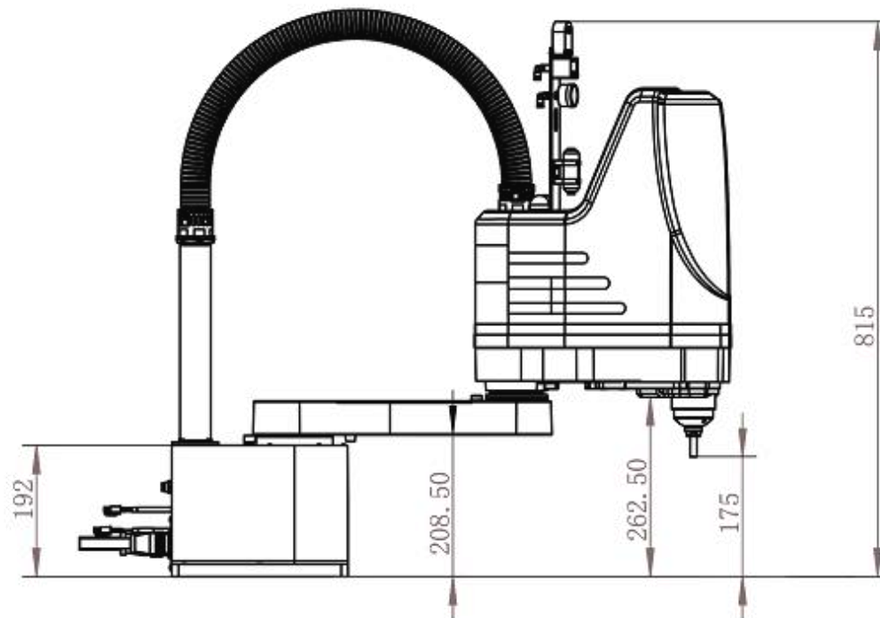
气吹式锁螺丝机器人 Air-blown screw locking robot
